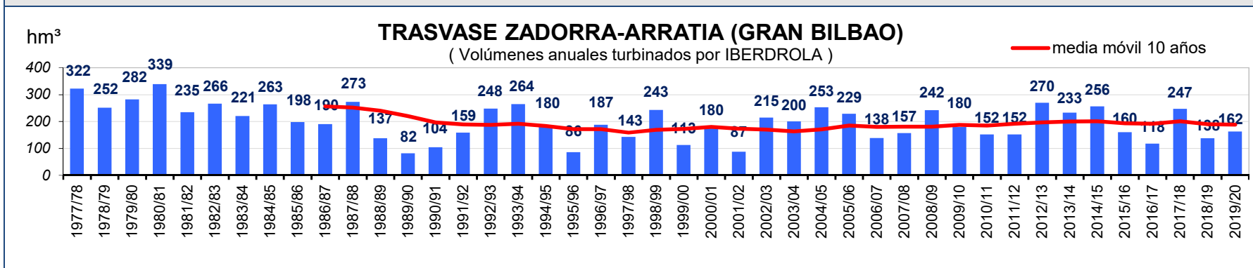
Figura 30. Evolución anual de los volúmenes transferidos: Traspase Zadorra-Arratia (Gran Bilbao)
