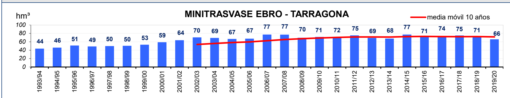
Figura 31. Evolución anual de los volúmenes transferidos: Minitrasvase Ebro-Tarragona
