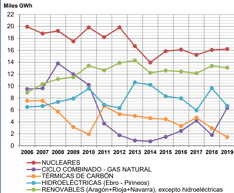
Figura 27. Evolución de la producción eléctrica anual en la demarcación hidrográfica del Ebro por fuentes (GWh) (2006-2019) (1)
