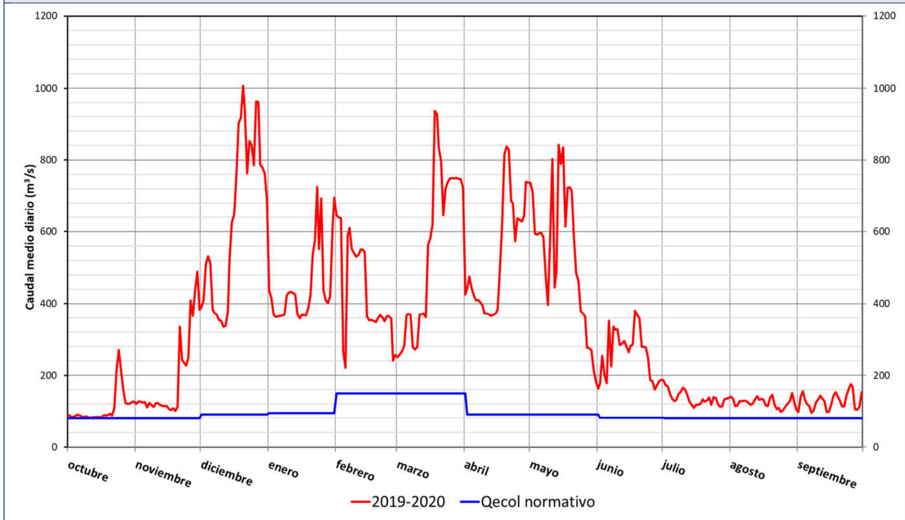
Figura 38. Hidrograma de la estación de aforos 027 Ebro en Tortosa año 2019-20 (caudales medios diarios) y el régimen de caudales ecológicos mínimos establecido en el Plan Hidrológico 2015-2021 (m 3 /s)
